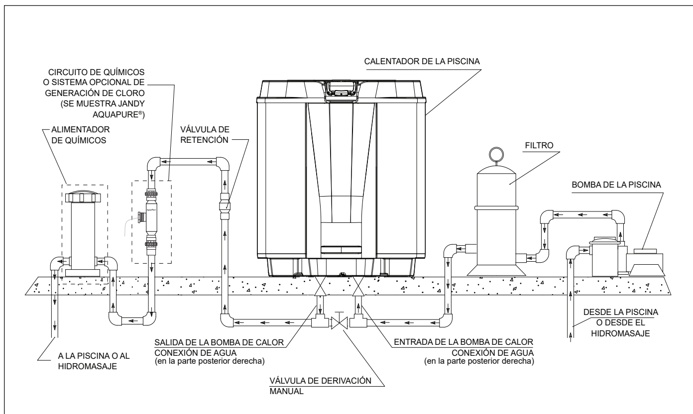
Figura 4. Disposición estándar de las tuberías
