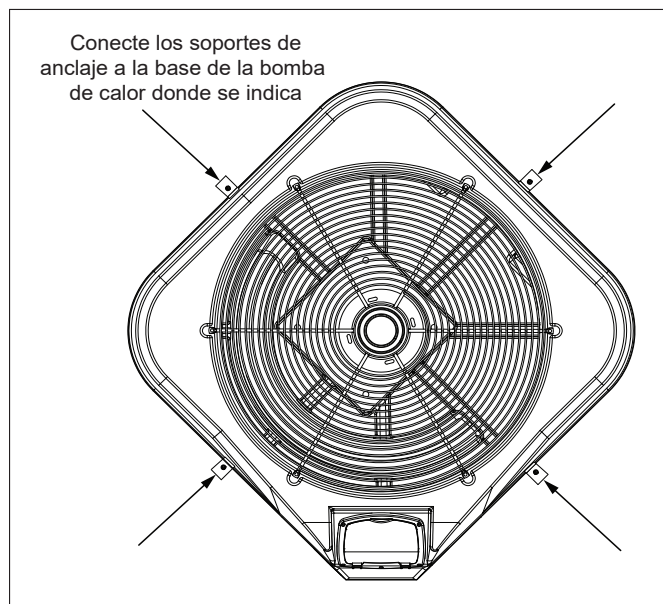
Figura 2. Posiciones de las abrazaderas de anclaje
