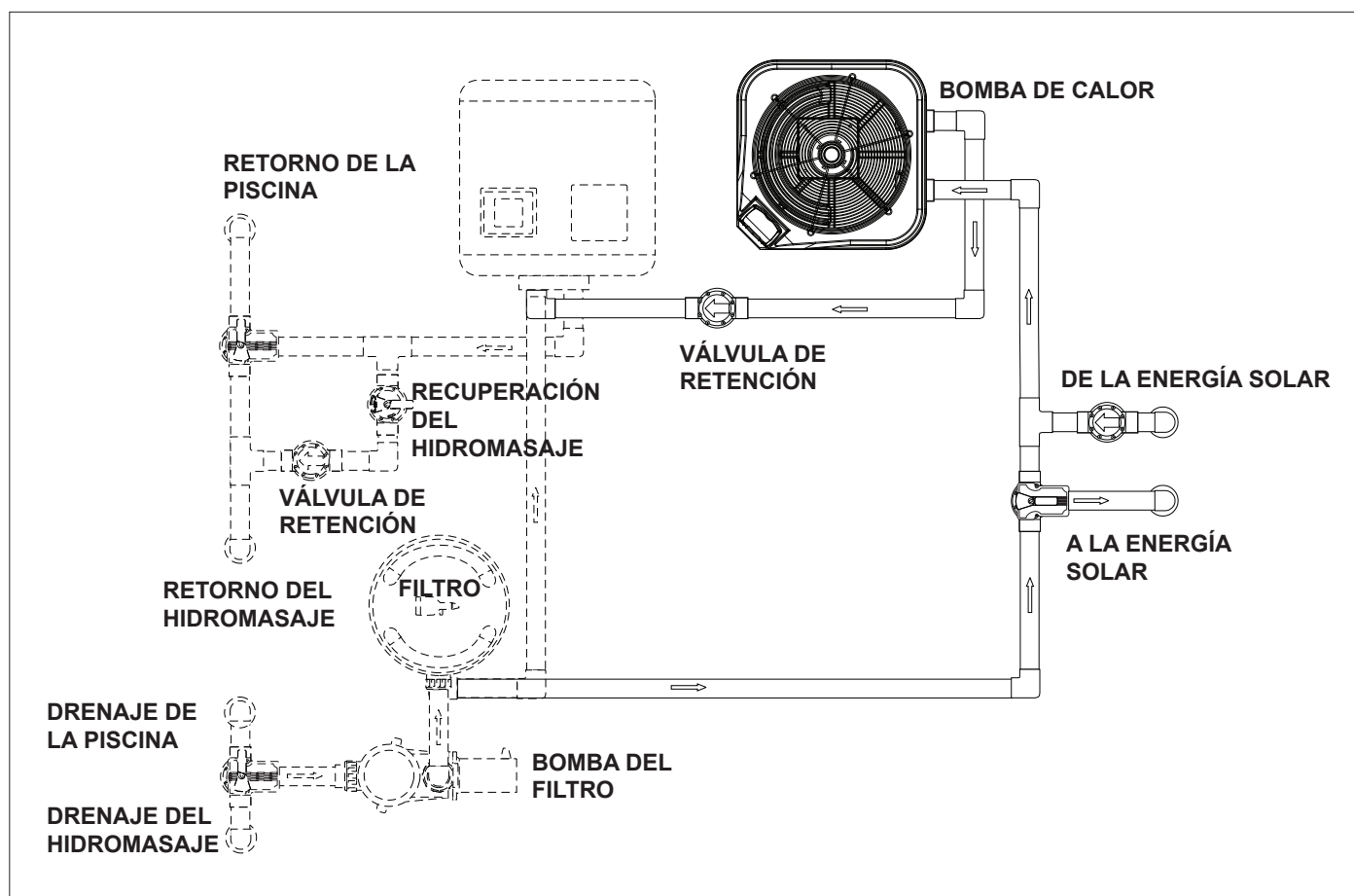
Figura 5. Tuberías para combinaciones de sistemas de calentamiento
