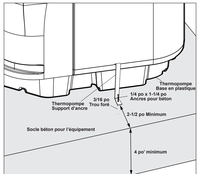
Figure 3. Installation de la bride d'ancrage
