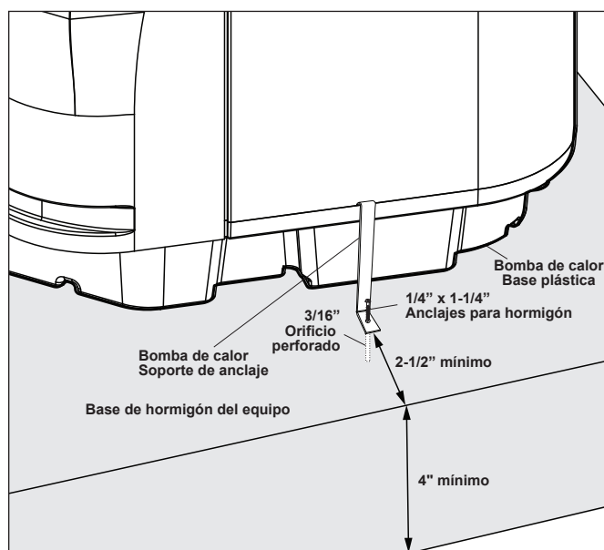
Figura 3. Instalación de las abrazaderas de anclaje
