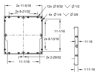
Part # R1216FR101 12 per case
