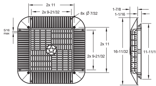
Part # 1216xxx
