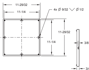
Part # 1216FR101 12 per case
